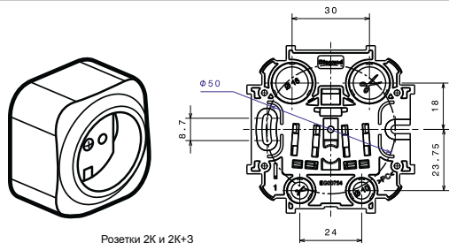
Розетки 2К и 2К+3 Кат. № 7 822 10 / 11 / 20
