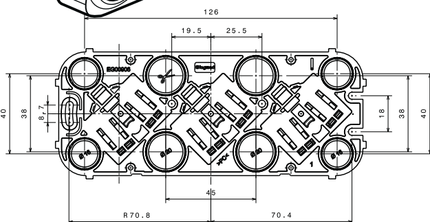
Розеточный блок x 3 Кат. № 7 822 18
