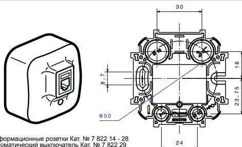
Информационные розетки Кат. № 7 822 14 - 28 Автоматический выключатель Кат. № 7 822 29
